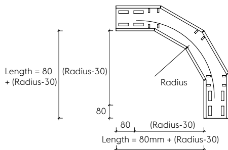
90° riser
